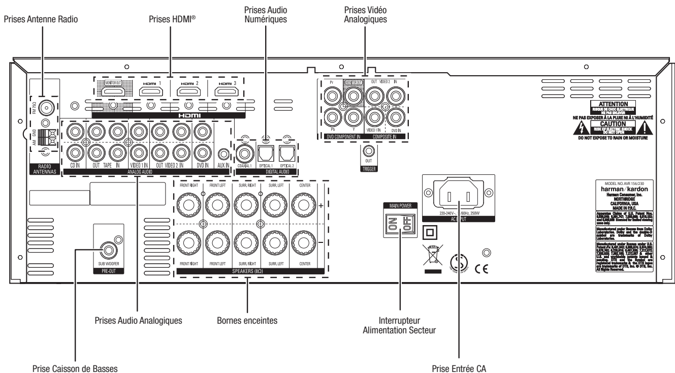
Raccordements au panneau arrière de l'AVR 156
